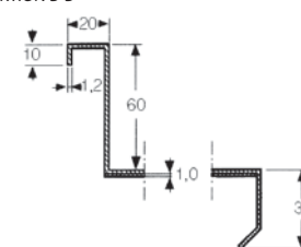
SEKTION B-B
